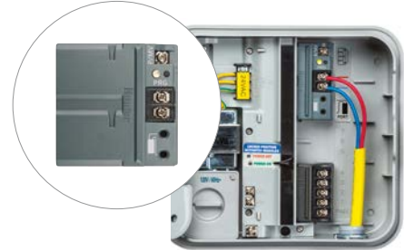
Pro-C ve HPC Kontrol Üniteleri için PC-DM Dekoder Çıkış Modülü
