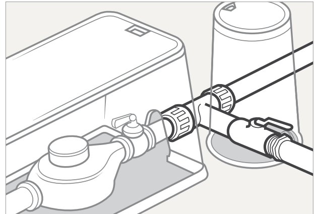
Miesto napojenia pri podnebí, kde nemrzne: Na pripojenie zavlažovacieho systému k vodovodnému systému v domácnosti použijete mosadzný kompresný T kus.
