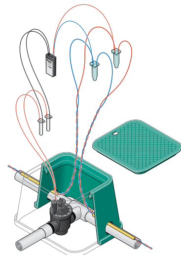
Câblage avec du mou pour la maintenance
